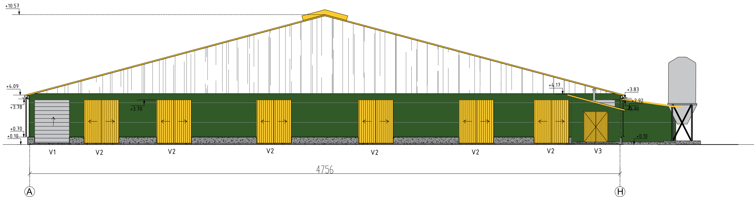
FASADAS TARP AŠIŲ A-H, M1:200
