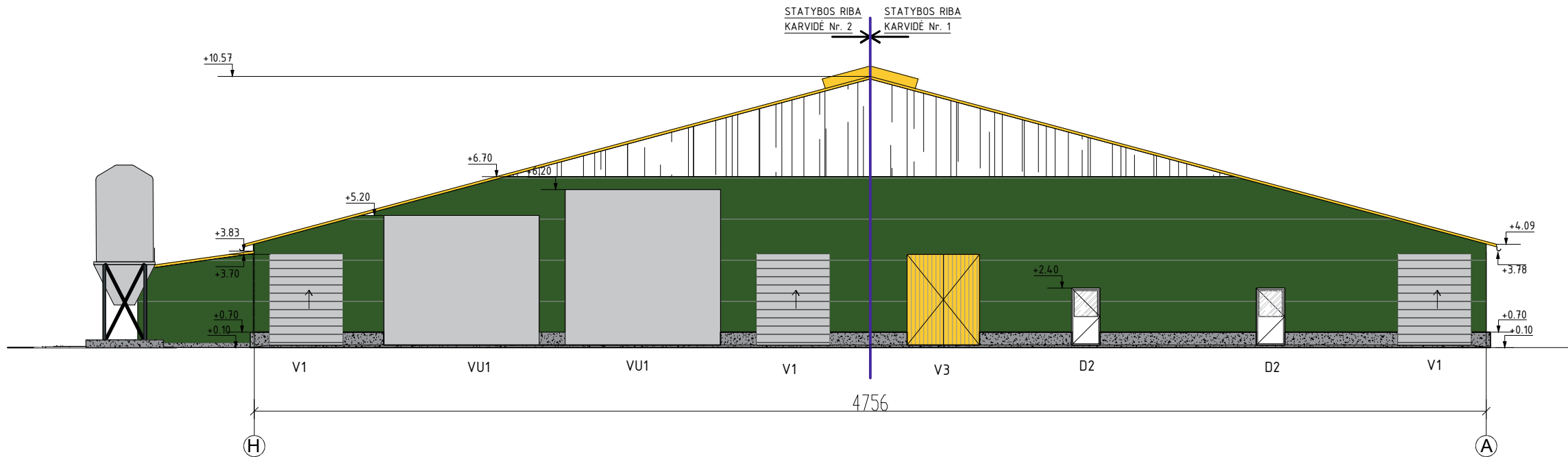
FASADAS TARP AŠIŲ H-A M1:200
