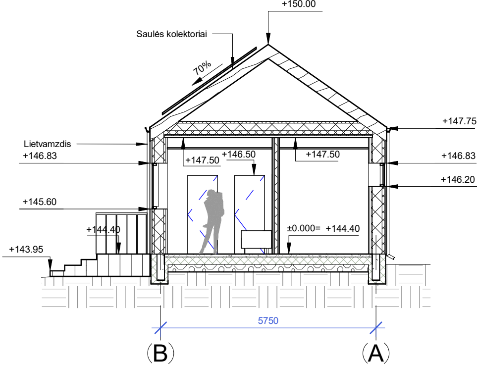
Pjūvis 2-2, M1:100
