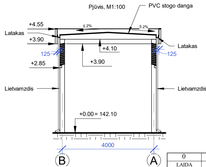
Pjūvis, M1:100
