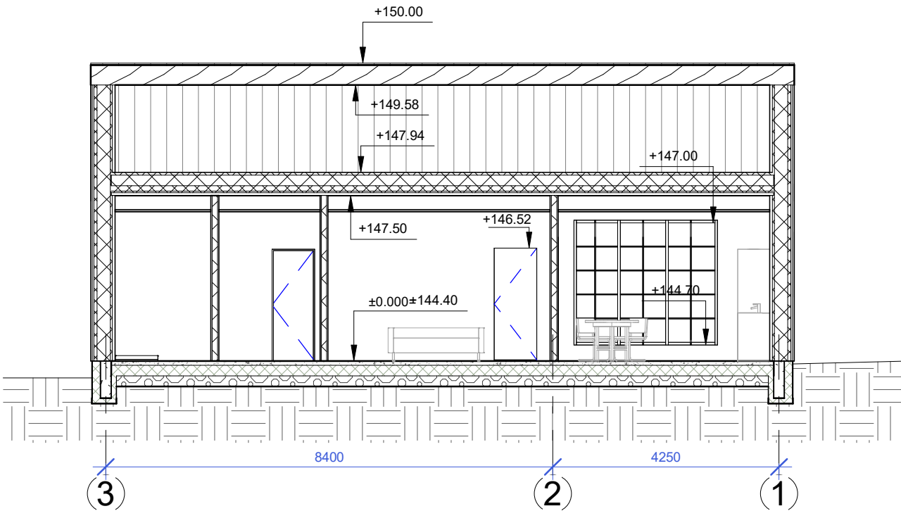
Pjūvis 1-1, M1:100
