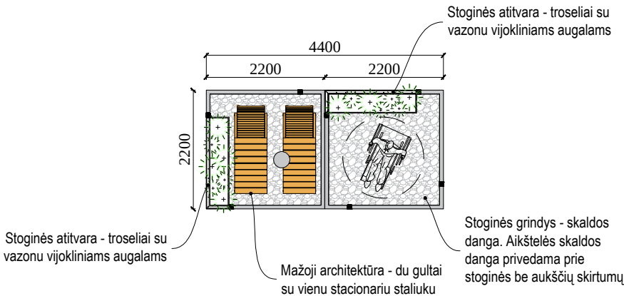
STOGINĖS STOTELĖJE NR. 2 PLANAS M 1:100
