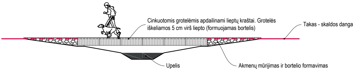
LIEPTO FASADAS
