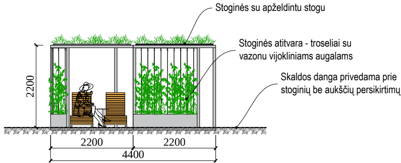
STOGINĖS STOTELĖJE NR. 2 FASADAS M 1:100
