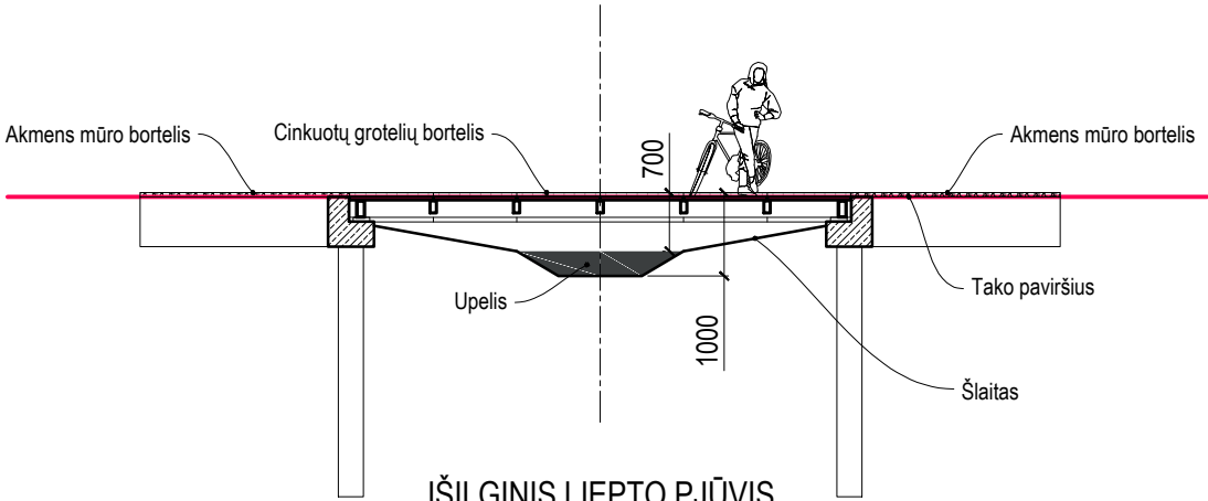
IŠILGINIS LIEPTO PJŪVIS
