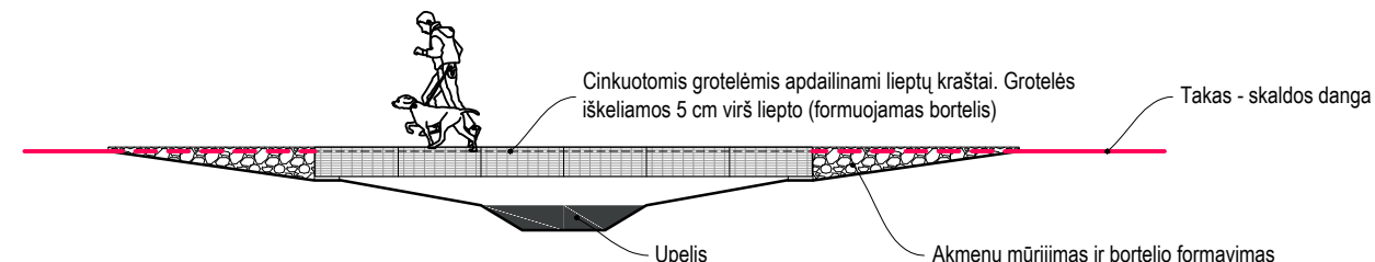
LIEPTO FASADAS
