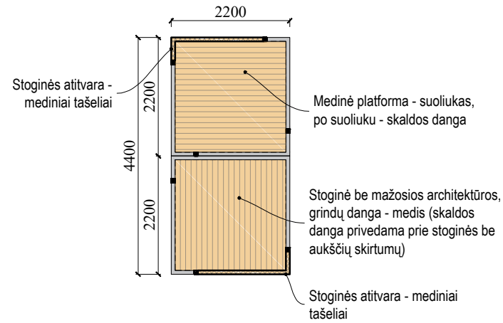
STOGINĖS VAISTAŽOLIŲ LAUKUOSE PLANAS M 1:100
