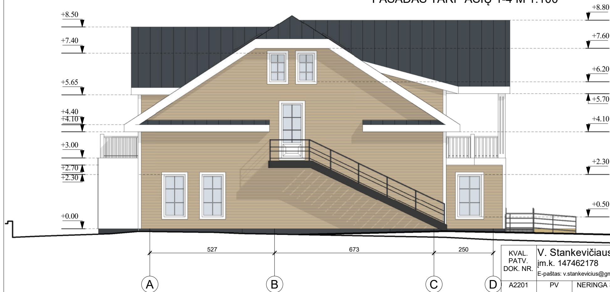
FASADAS TARP AŠIŲ A-D M 1:100
