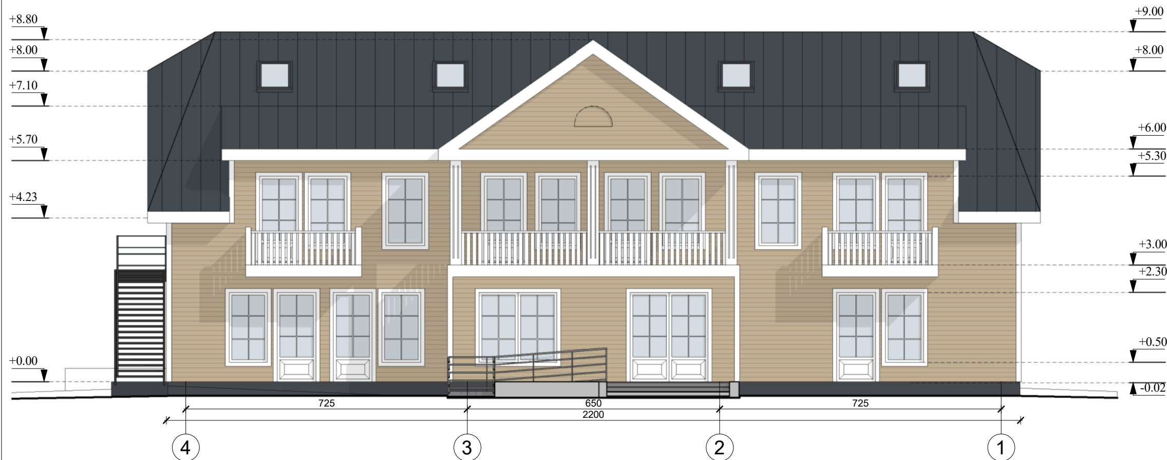
FASADAS TARP AŠIŲ 4-1 M 1:100
