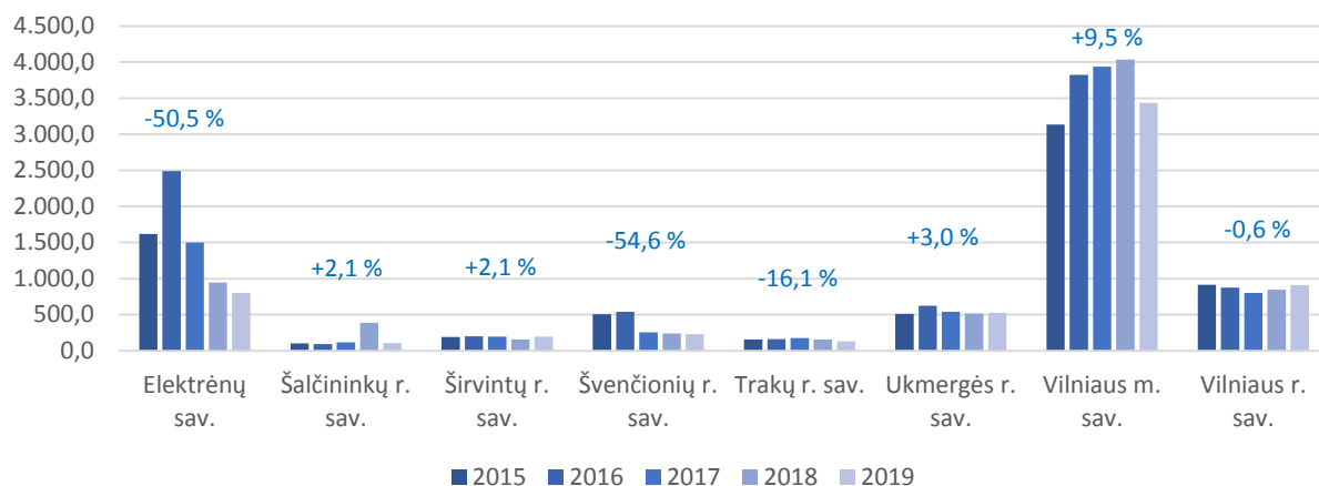
2.5.1.2. pav. Teršalų, išmestų į aplinkos orą iš stacionarių taršos šaltinių, kiekis 2015–2019 m. (t) ir jo dinamika 2015–2019 m., proc.
